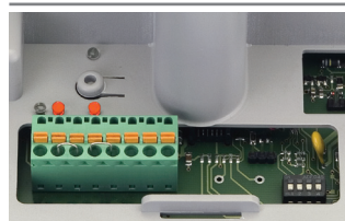
Scheda elettronica E 600 incorporata
