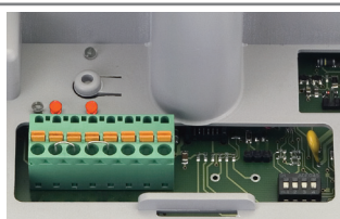
Scheda elettronica E 1000 incorporata
